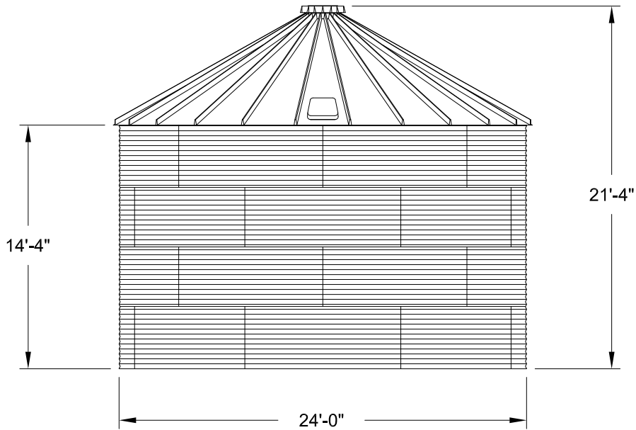
ELEVATION
