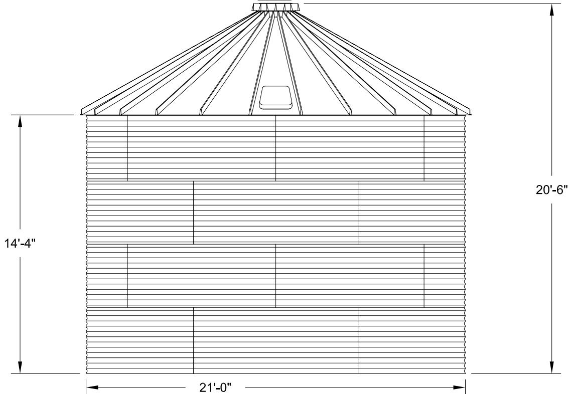
ELEVATION
