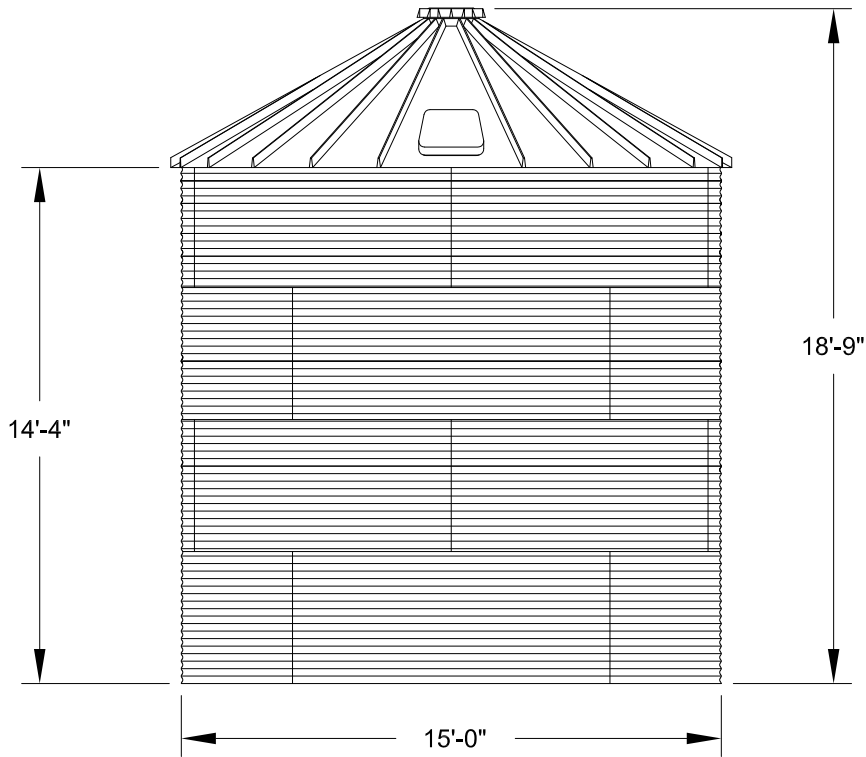
ELEVATION
