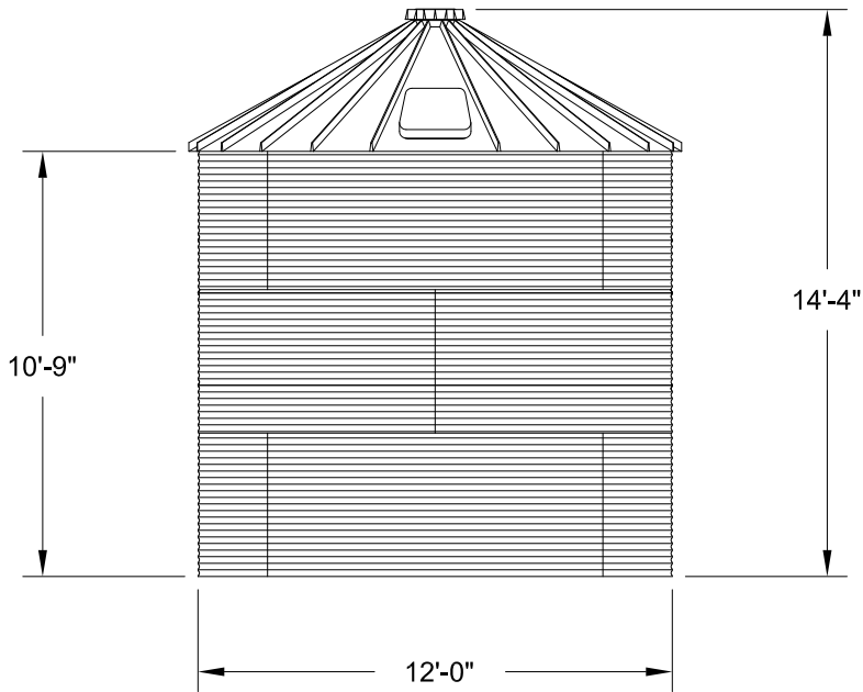
ELEVATION
